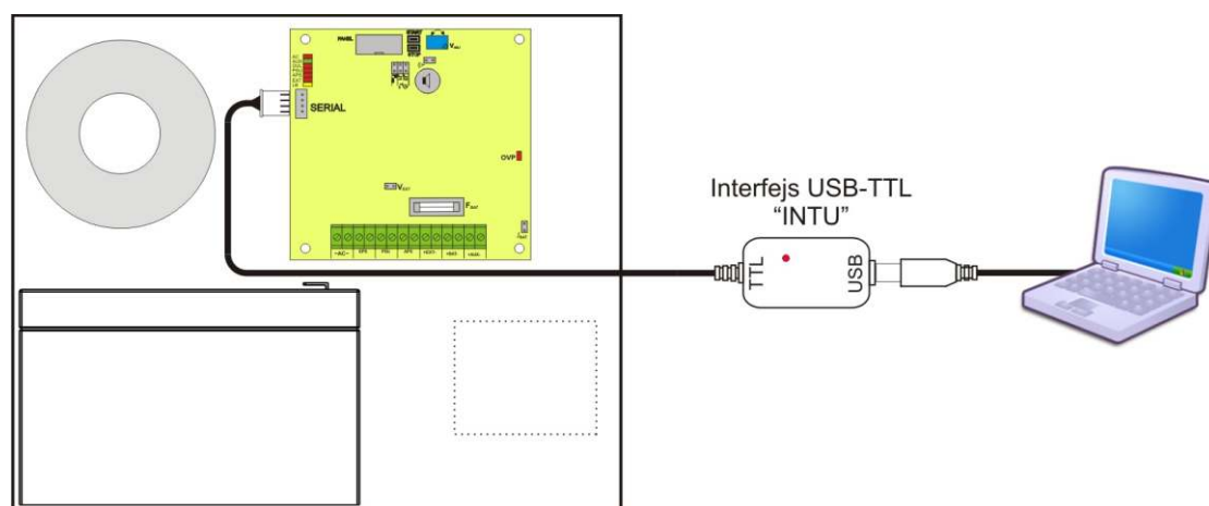
Komunikacja USB-TTL z wykorzystaniem interfejsu USB-TTL „INTU”.
