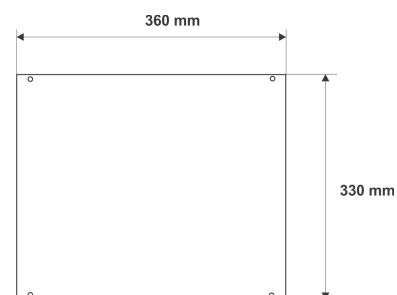
blacha montażowa
